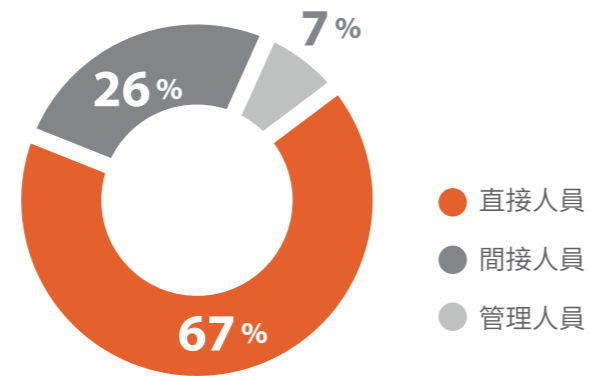
直接比例
